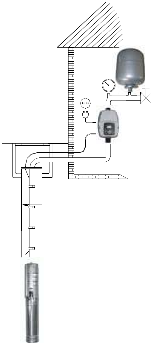
Sposób instalacji przetwornicy częstotliwości.
